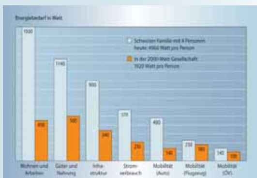
Energiebedarf einer Familie mit 4 Personen – heute und in der 2000 - Watt - Gesellschaft
